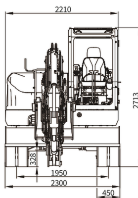
FRONTANSICHT
