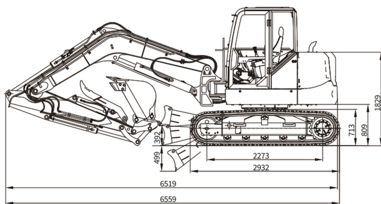
SEITENANSICHT
